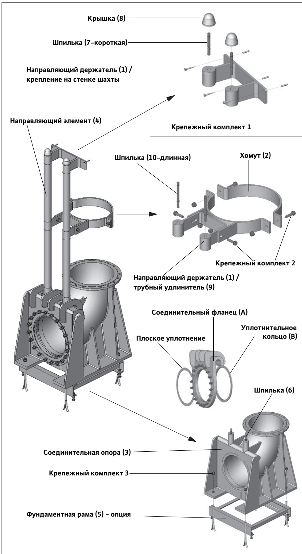
Рис. 1-6: Монтаж устройства подвески
